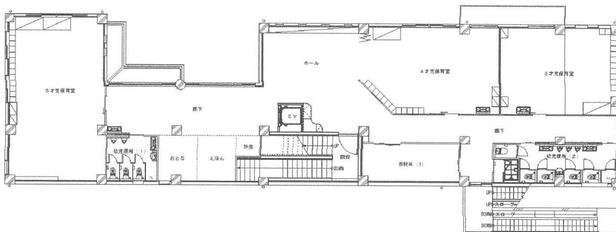
(3階)
